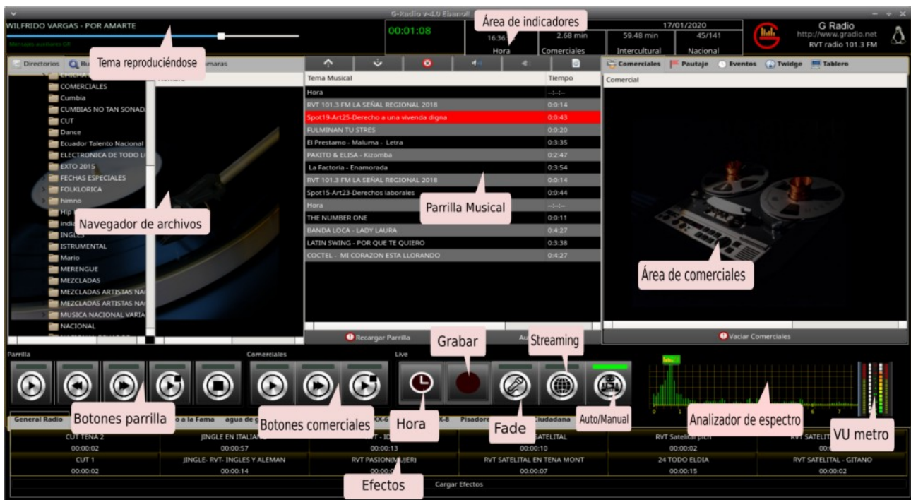
Ilustración 19: Interfaz Principal de G-Radio
