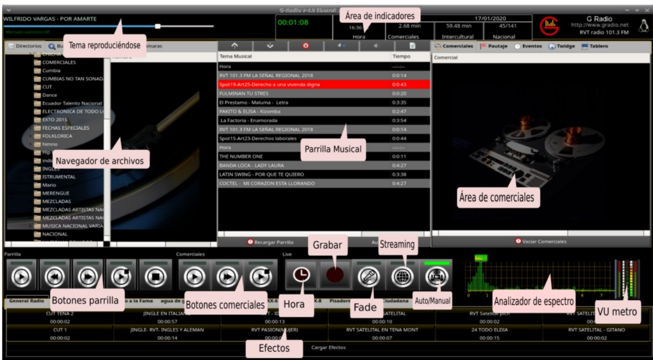
Ilustración 1: Interfaz principal de G-Radio y sus principales funciones
